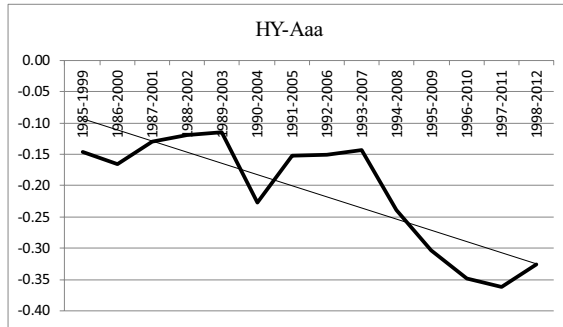
(b) HY-Aaa
