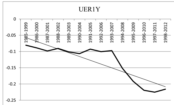
(d) UR
